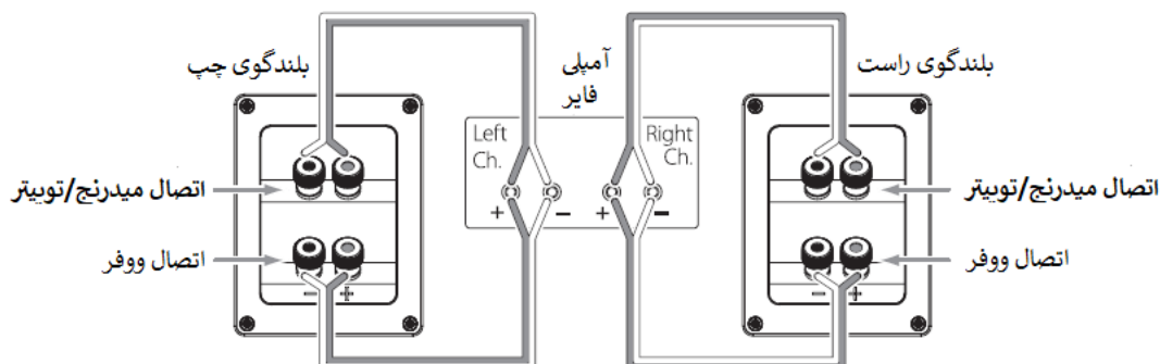
آمپلی فایر تک دو سیمه
