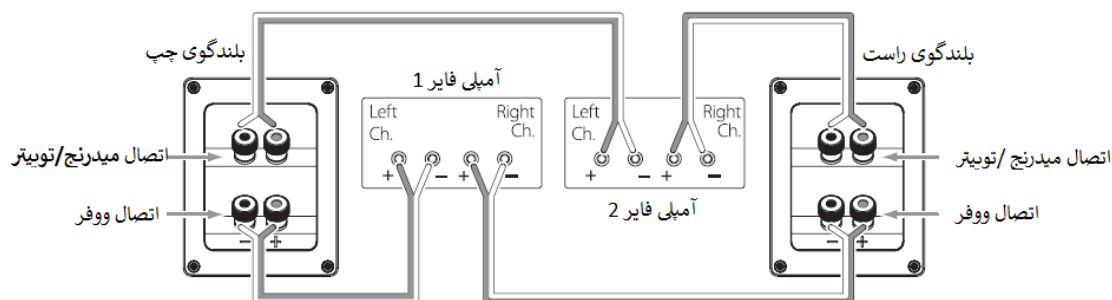
آمپلی فایر دوتایی دو سیمه
